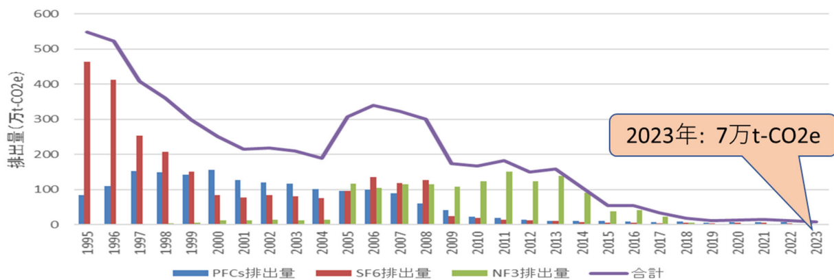
製造プロセスで排出されるPFCs、SF 6 、NF 3 の推移
